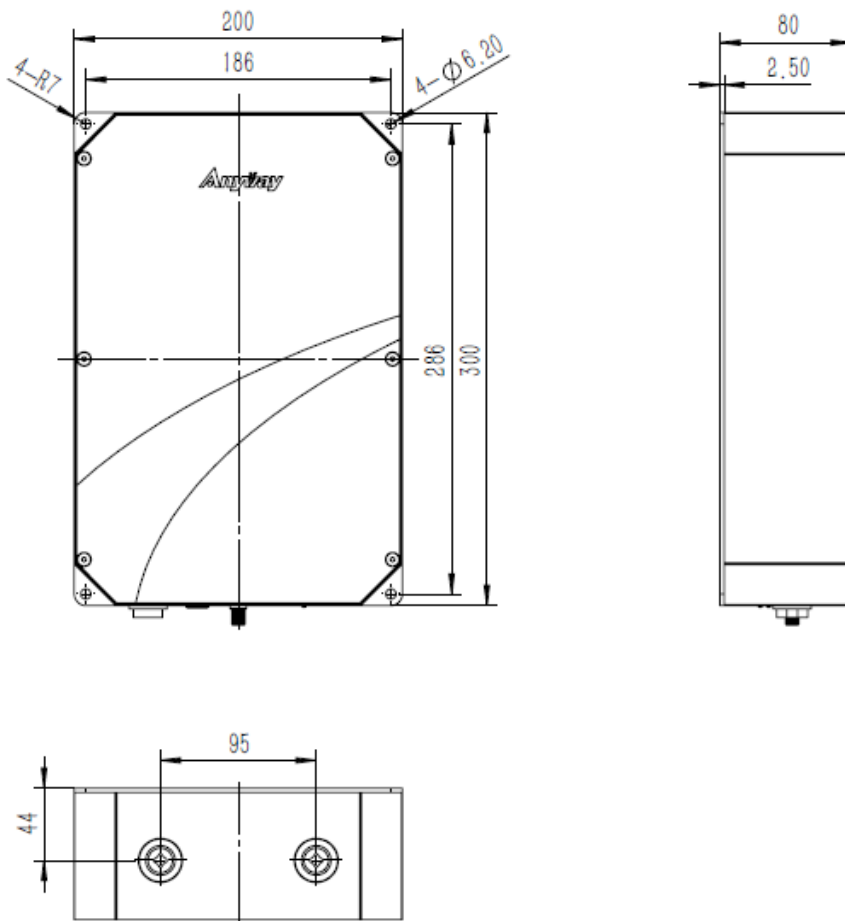
图 1 外形尺寸图
